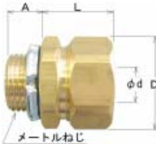
RBC 形 ストレートコネクタ
