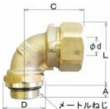
RLC 形 90° コネクタ
