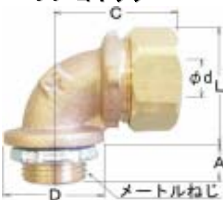
RBC 形 90°コネクタ
