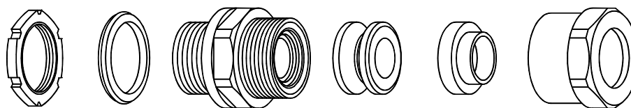
ロックナット (鋼) ボディパッキン (NBR) ニップル (ZDC2) シールブッシング (NBR) テ-パ-ワッシャ (141766) 締付ナット (ZDC2)
