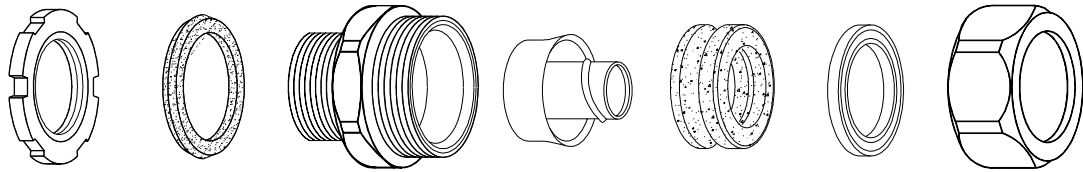
ロックナット (鋼製) ボディパッキン (NBR) ニップルボディ (C3604) ターミナルキャップ (SPCC) シールグランド (NBR) Uスリーブ (POM) ジャムナット (C3604)
